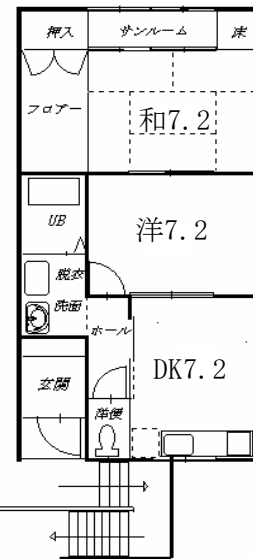
間取 102号室
